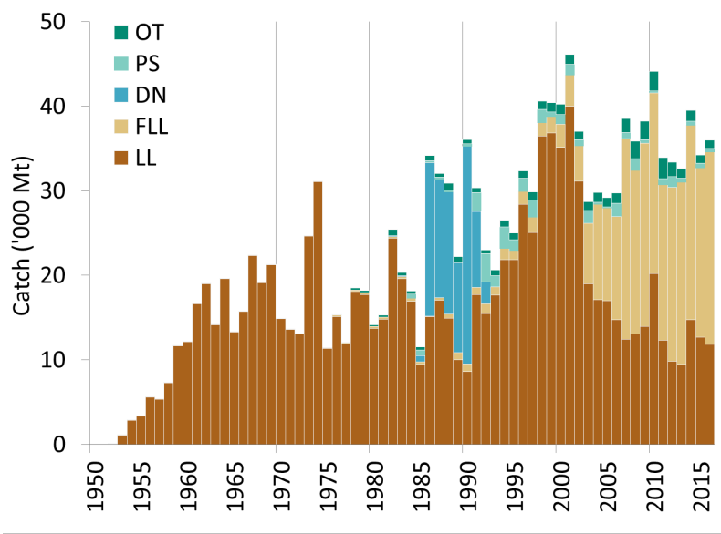
Figure 1. Germon : Prises de germon par engins (données 1950-2016).
